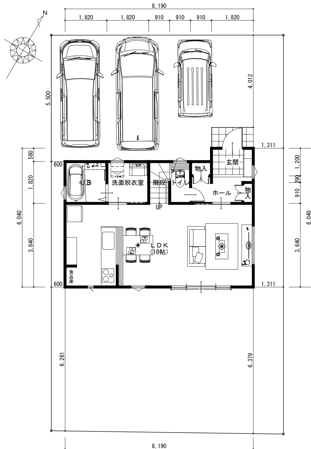
1階 平面図 S:1/100
