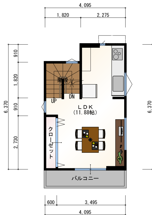
2階 平面図 S:1/100
