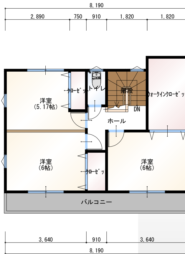
2階 平面図 S:1/100
