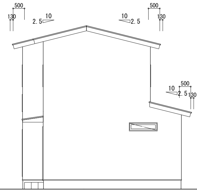
東側 立面図 S:1/100
